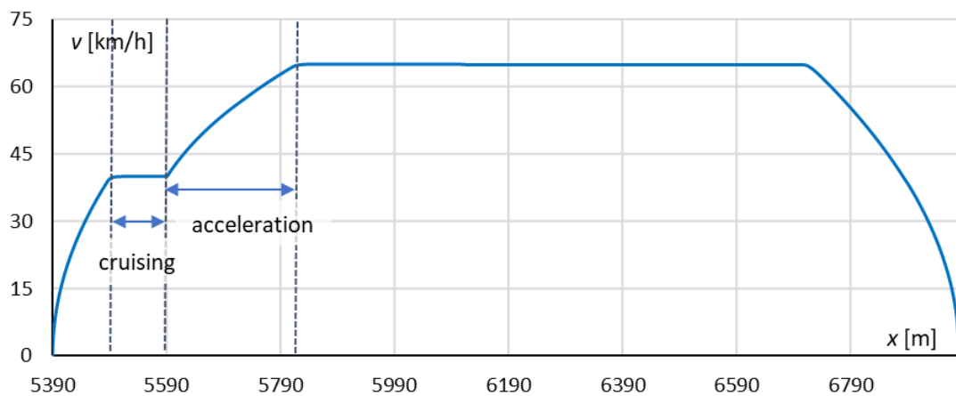
Fig. 5.43. Example of irregular velocity profile – local limit on pedestrian crossing (Gdańsk Zaspą – Gdańsk Przymorze, track 501, direction →Gdynia)
