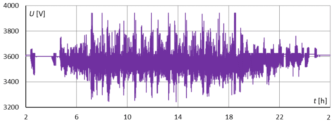
Output voltage – substation Gdańsk Wrzeszcz (optimized run)
