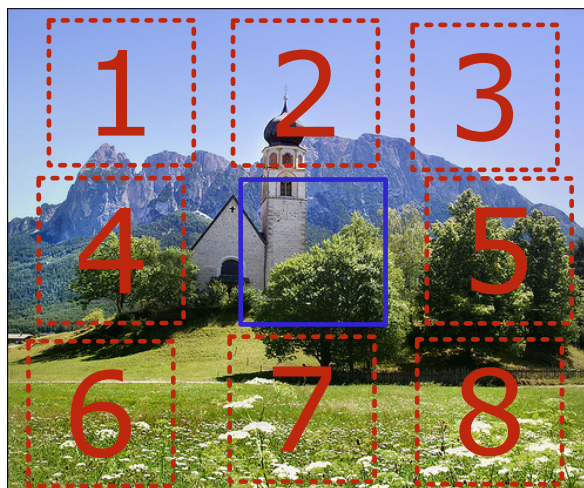
Rysunek 6.3: Metoda przewidywania relacji pomiędzy fragmentami obrazu
