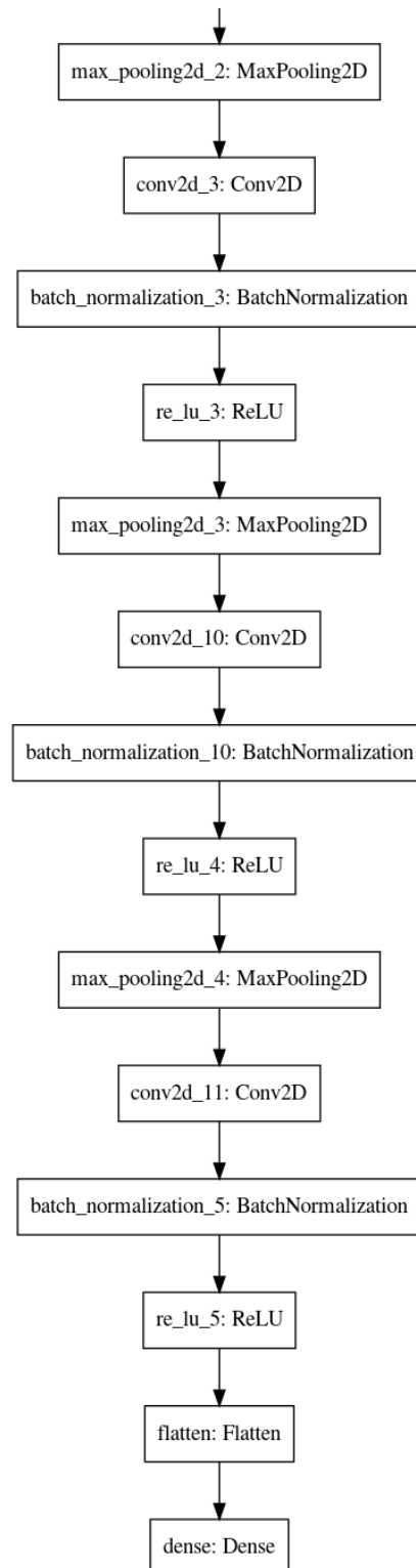
Rysunek 5.8: Schemat struktury otrzymanej w wyniku działania algorytmu: sieć 4 – część 2
