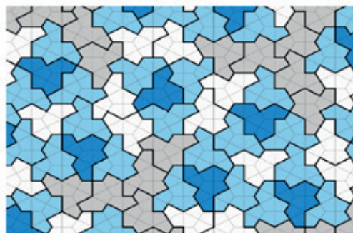
Rys. 5. Pierwszy parkietaż einsteinowski odkryty w 2023 roku
