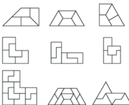
Rys. 4. Parkietaże samopowielające się
